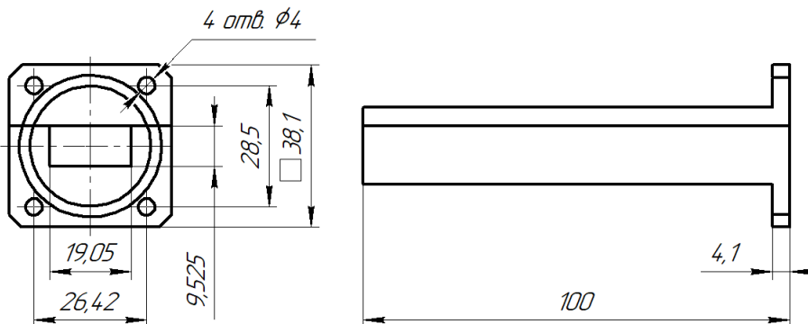
Рисунок 1 – Общий вид и габариты изделия.
